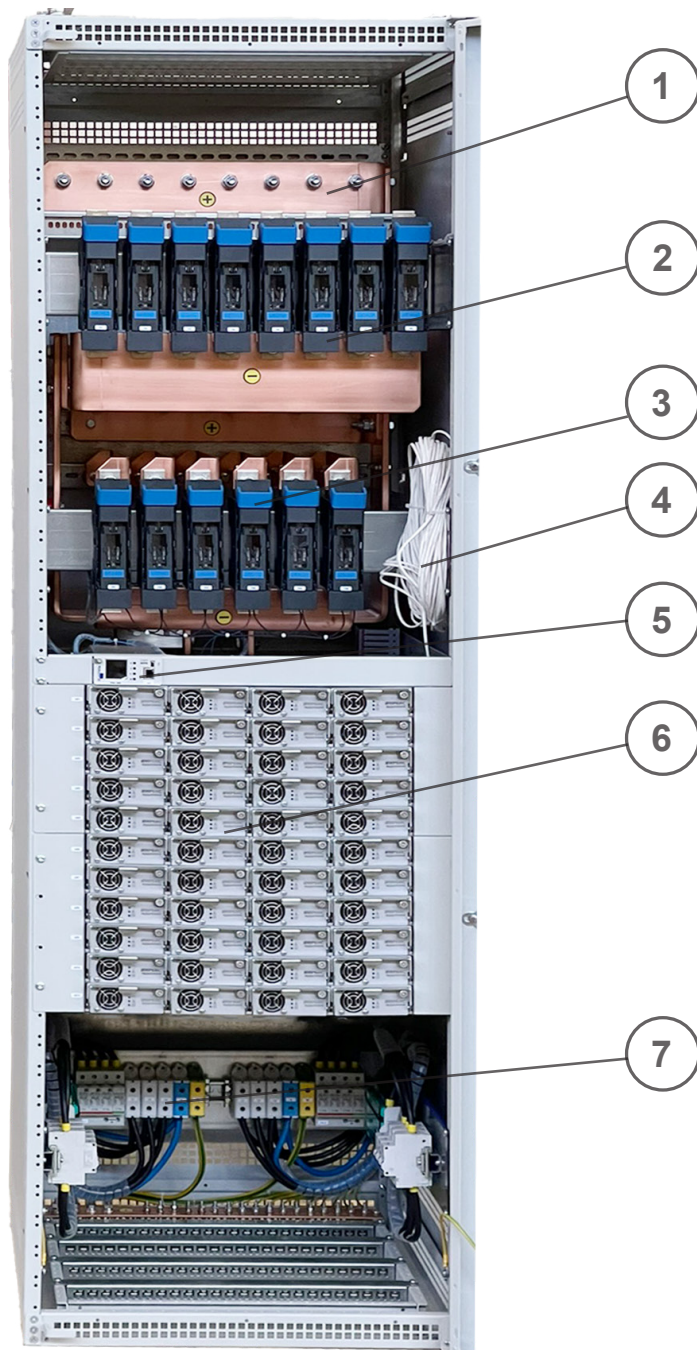
Рисунок 1.1 - Электропитающая установка ИрДи PS48
