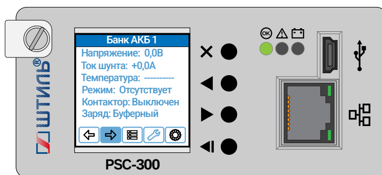
Рисунок А4 - окно « Банк АКБ1»
