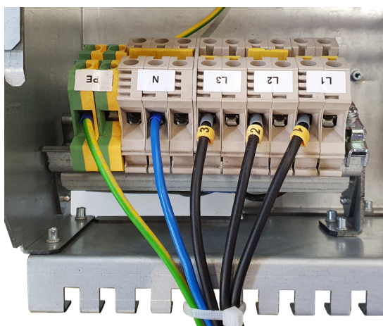
Рисунок Б1.2. Подключение и фиксация кабелей
