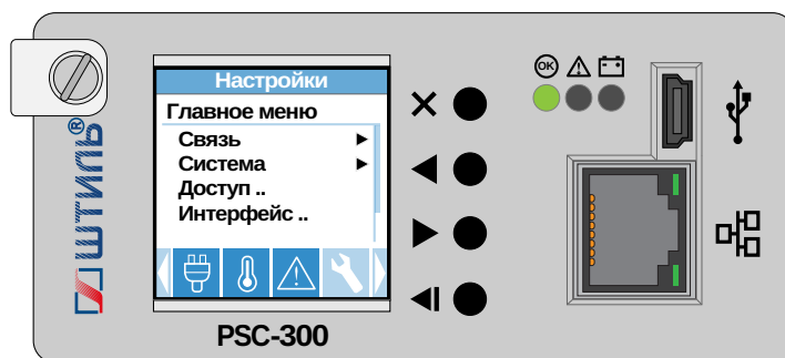
Рисунок 2.1 – Лицевая панель контроллера Штиль PSC-300
