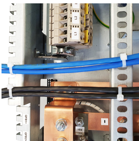
Рисунок Б2.4. Фиксация на задней стенке
