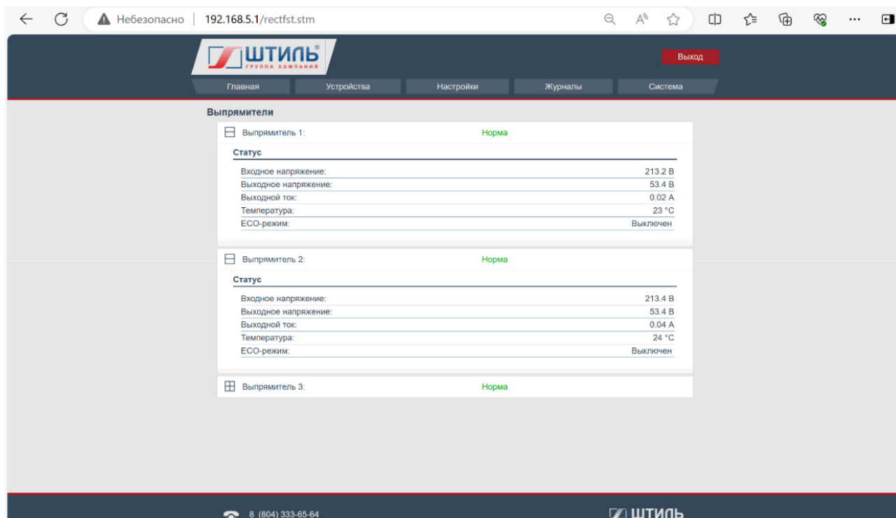
Рисунок А51 - Параметры работы каждого выпрямителя системы питания отдельно
