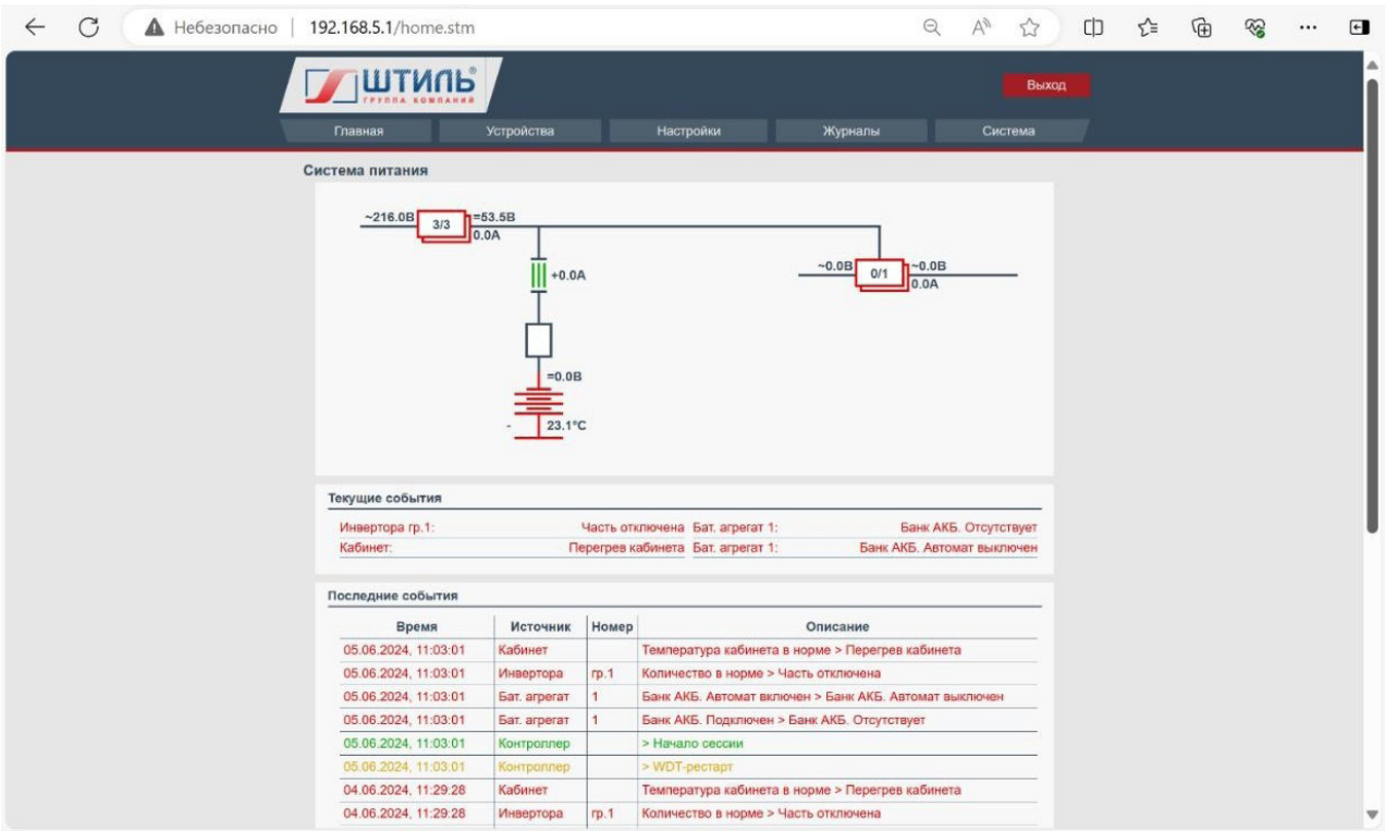
Рисунок А3- Главная страница WEB- интерфейса мониторинга и управления
