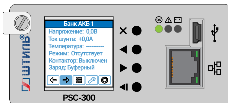
Рисунок А4 - окно « Банк АКБ1»
