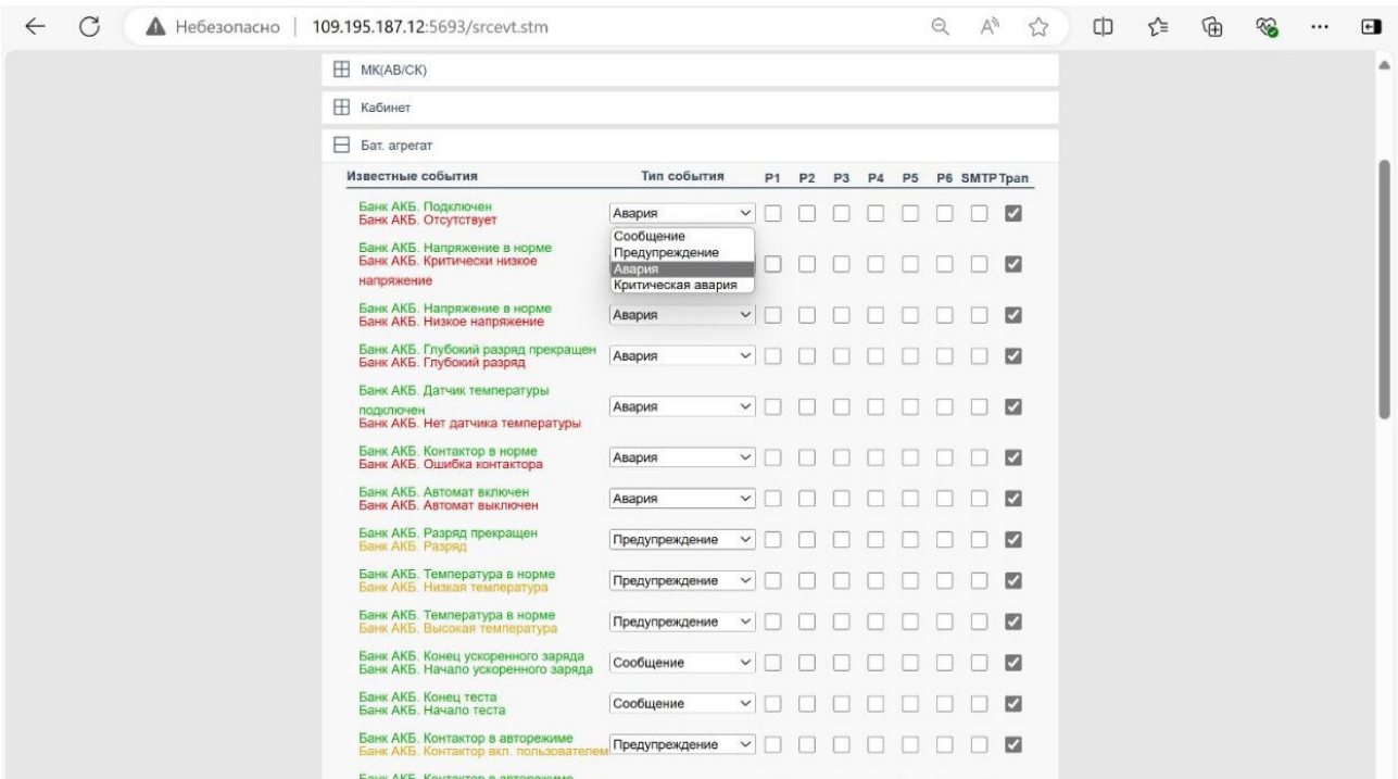
Рисунок A25 - Настройка параметров приоритетов аварий батарей
