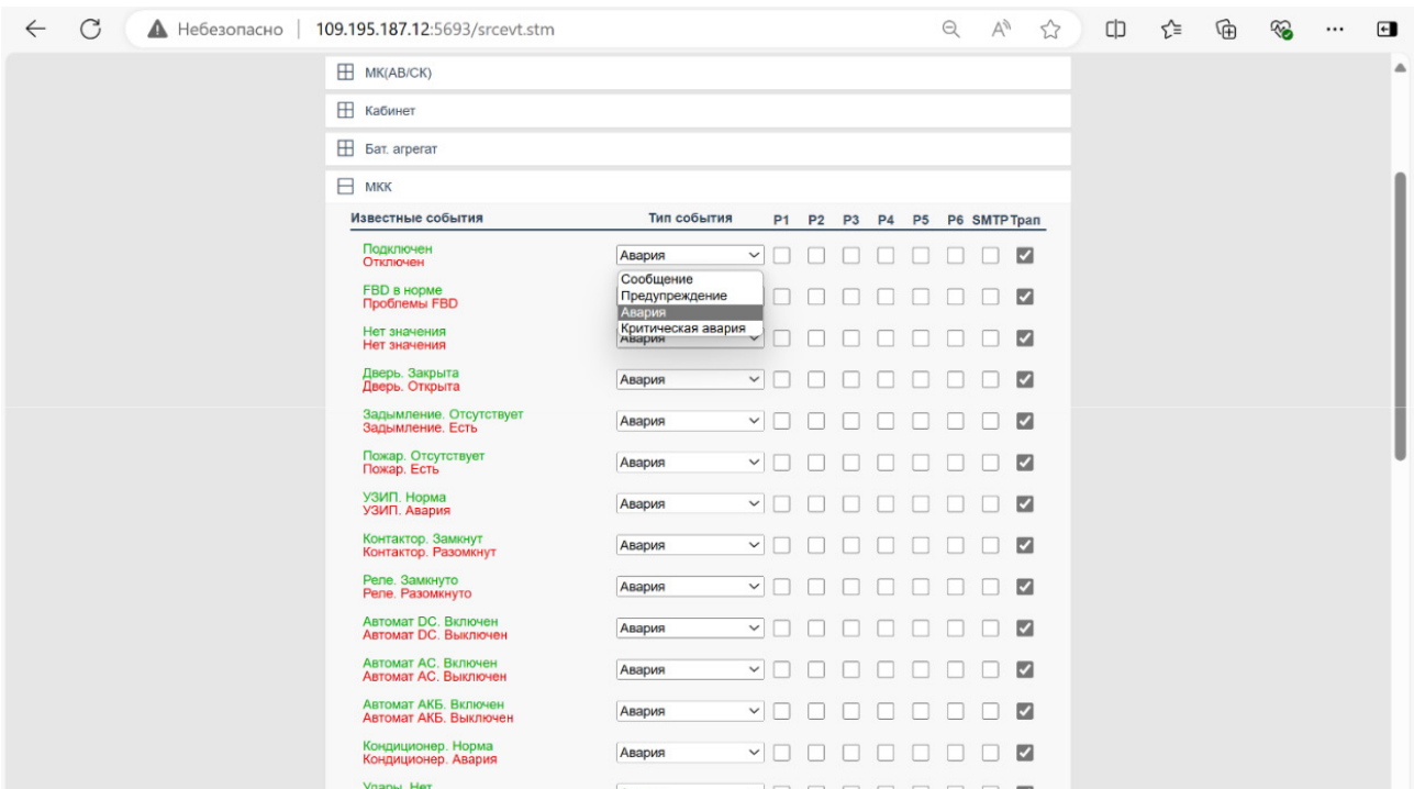
Рисунок A26 - Настройка параметров приоритетов аварий МКК
