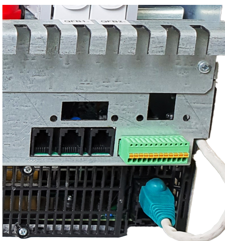
Рисунок Б4.2. Подключение сигнальных контактов
