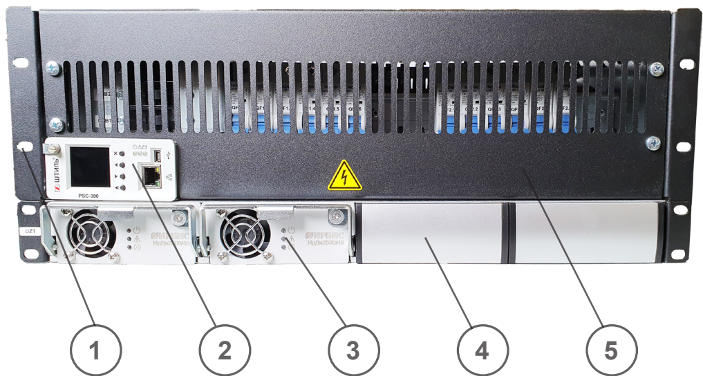
Рисунок 1.1 - Электропитающая установка ИрДи PS48 10 кВт 4U
