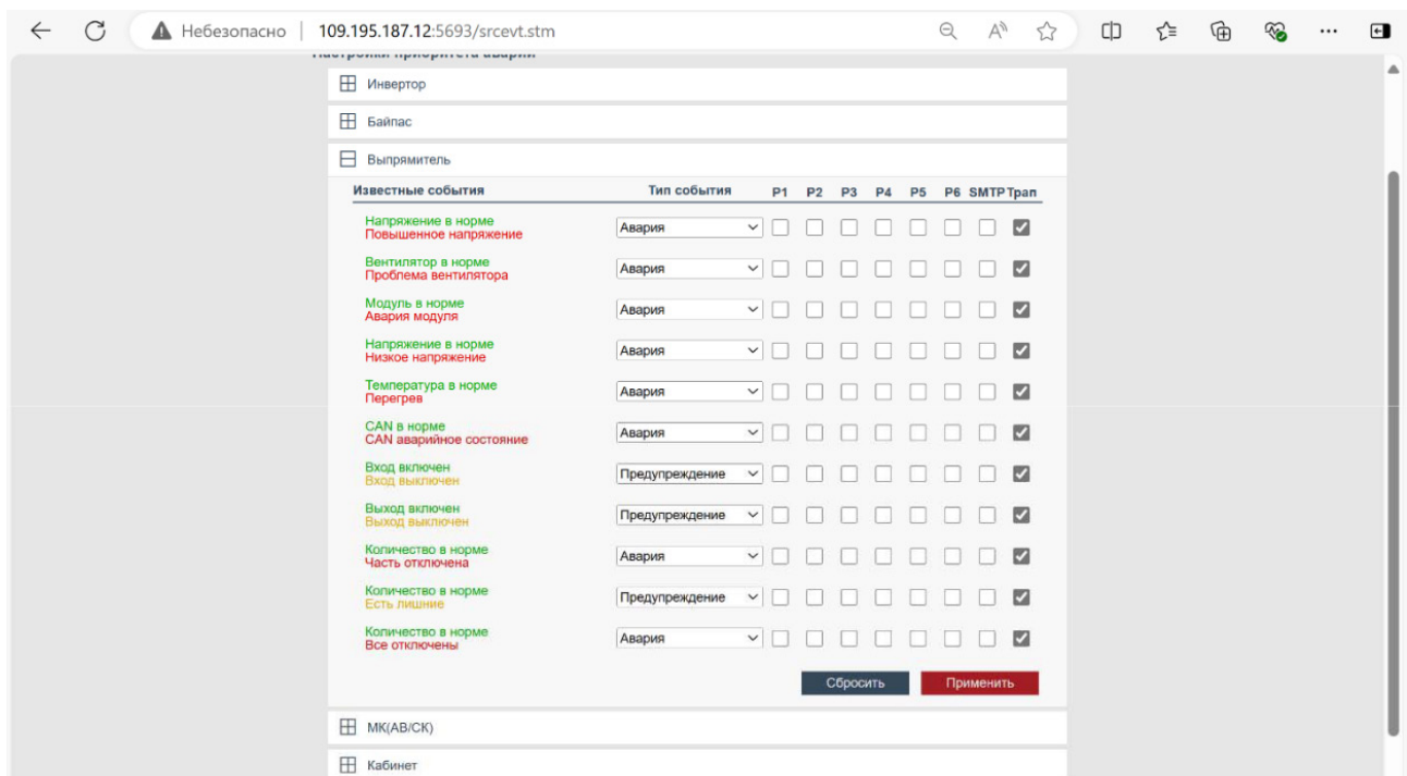
Рисунок A22 - Настройка параметров приоритетов аварий выпрямителя
