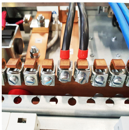
Рисунок Б2.2. Подключение «плюса» нагрузки
