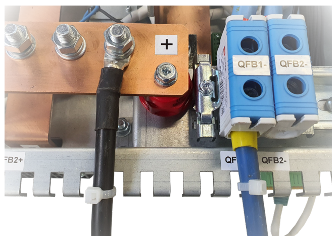
Рисунок Б3.2. Подключенные кабели АБ
