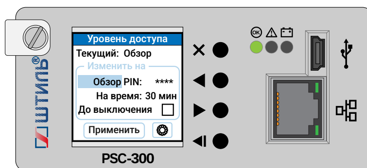
Рисунок А16 - Окно «Уровень доступа»
