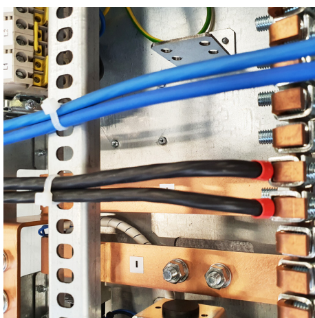
Рисунок Б2.3. Фиксация на кабельном держателе
