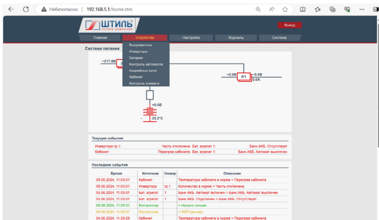
Рисунок А49 - Меню раздела «Устройства» WEB- интерфейса мониторинга
