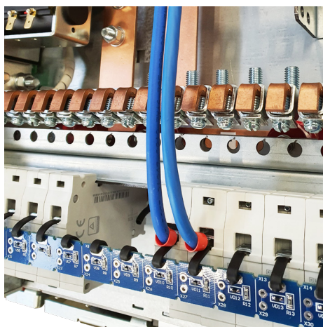
Рисунок Б2.1. Подключение «минуса» нагрузки
